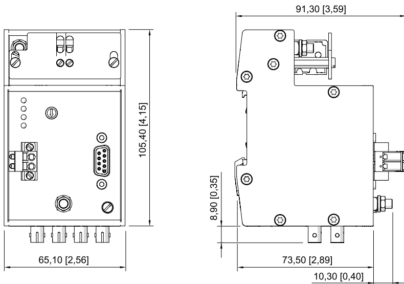
Medienkonverter 9786
