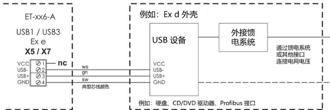
类型 2 接线图 (例如：硬盘、带 SV 的 CD/DVD)
