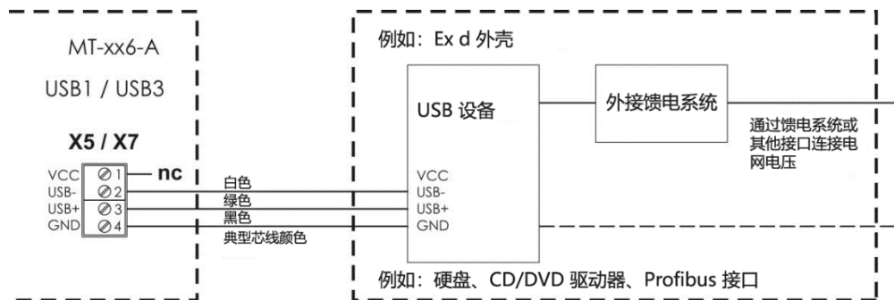
类型 2 接线图 (例如：硬盘、带 SV 的 CD/DVD)
