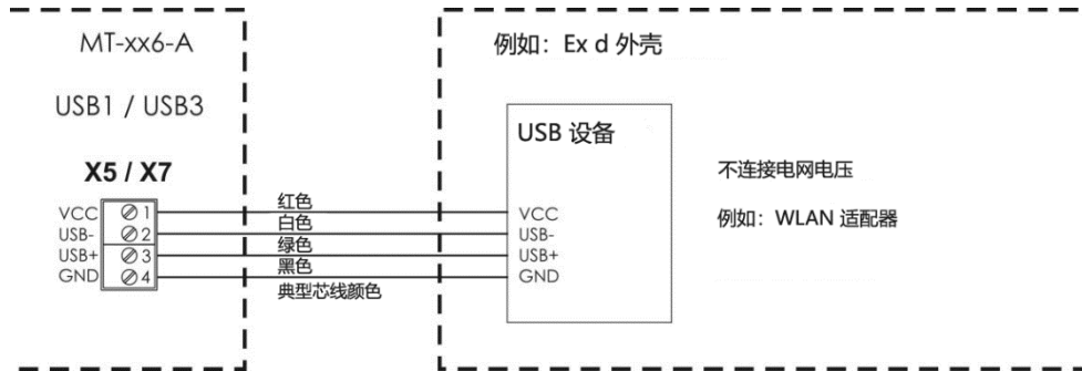
类型 1 接线图 (例如：WLAN 适配器)
