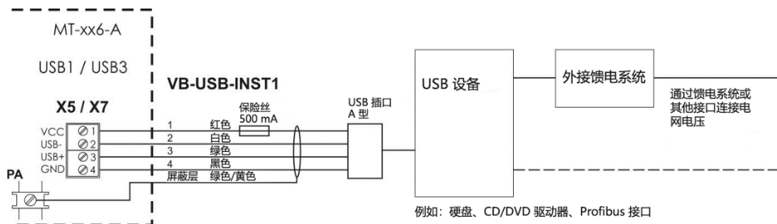
使用 VB-USB-INST1 是的连接图 (硬盘、带 SV 的 CD / DVD)
