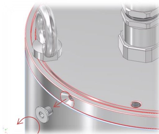
Fig.6-5: Remover o parafuso de embeber de tipo T08-TNXCD
