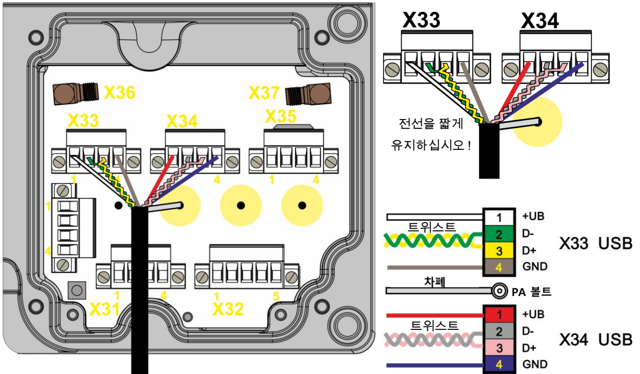
핀 할당 상세도
