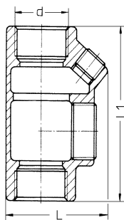
Zündsperrn Reihe EYS 5 ... 8
