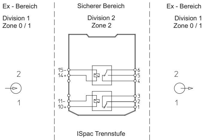
Anschlussplan 9172/22-11-00
