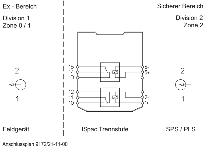
Anschlussplan 9172/21-11-00
