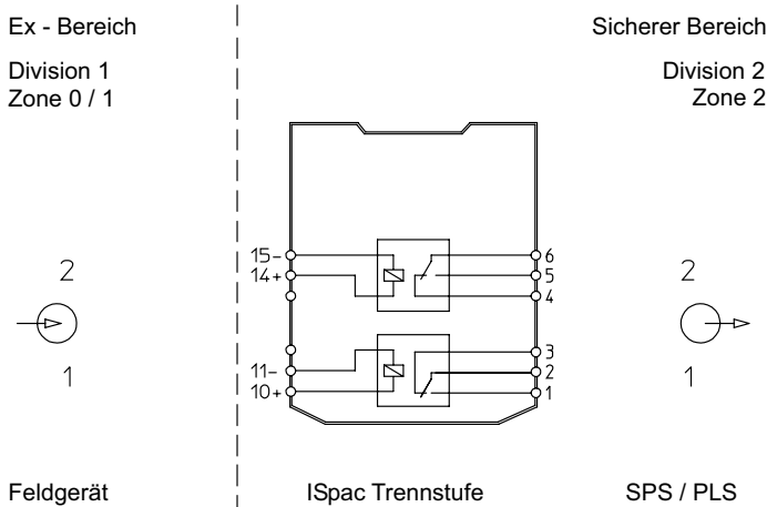
Anschlussplan 9172/20-11-00
