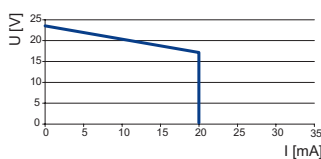
Ausgangskennlinie 9475/32-08-62, 9475/33-08-60
