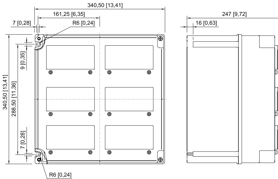
Gehäuse 8146/5086 für Akku-Kasten 8316/22-12-0250-1 für Akku-Kasten 8316/22-12-0400-1 für Akku-Kasten 8316/22-12-0600-1
