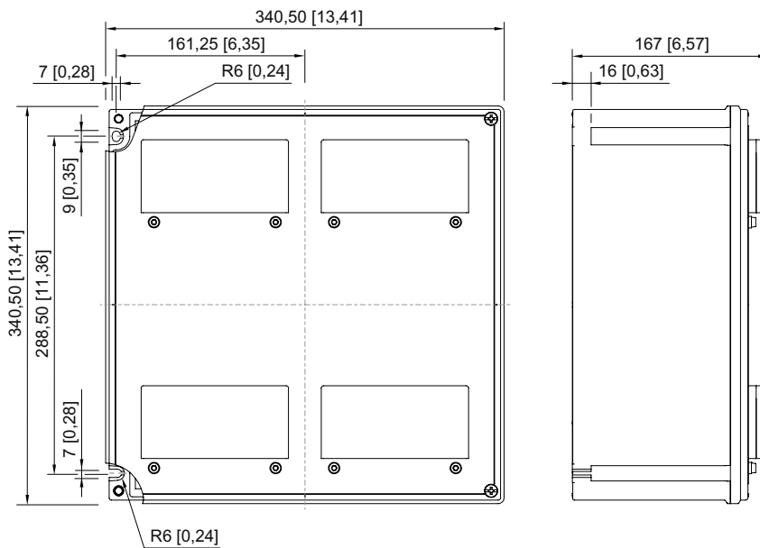
Gehäuse 8146/5083 für Akku-Kasten 8316/22-24-0100-1
