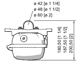
Rohrschelle montiert in Montageschiene
