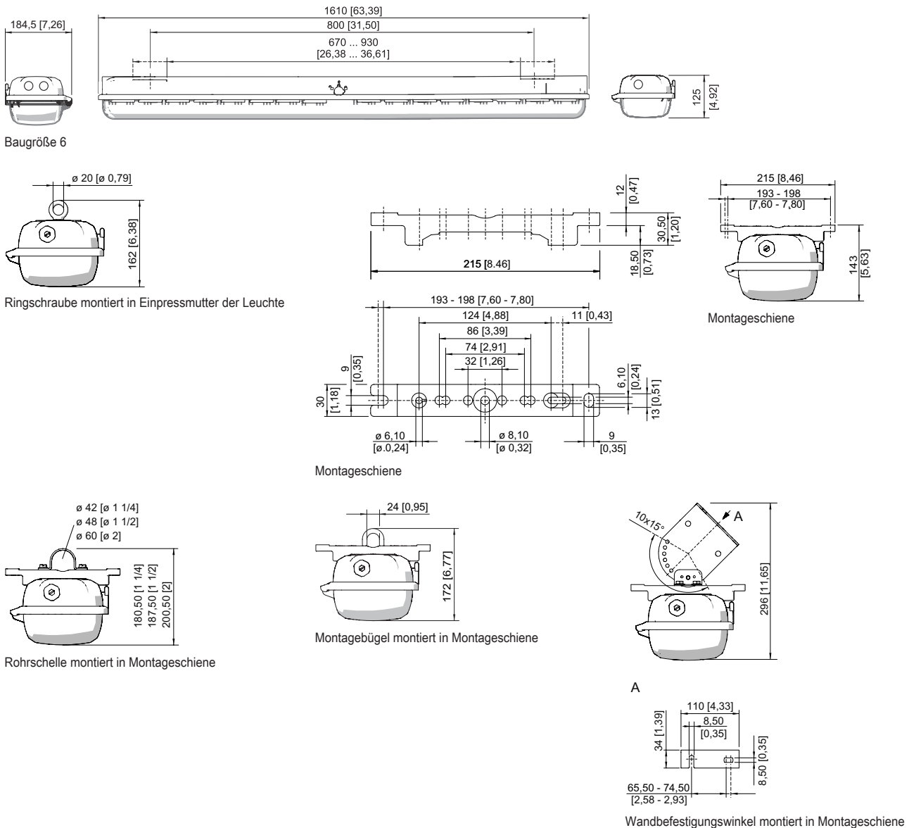
Wandbefestigungswinkel montiert in Montageschiene
