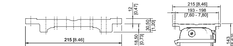
Montageschiene
