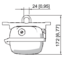
Montagebügel montiert in Montageschiene
