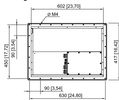
Schalttafel-Einbaumodul Rückansicht
