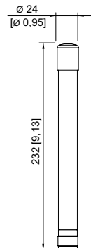
Antenne Typ 9790/1-2458-NTM-53
