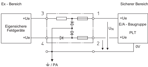
Zwei-Kanal-Sicherheitsbarrieren Sicherheitsbarriere Potential: + / Auswertebarriere Potential: +
