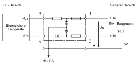
Zwei-Kanal-Sicherheitsbarrieren Sicherheitsbarriere Potential: + / Auswertbarriere Potential: +
