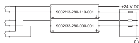
Anwendungsfall: Kombination von potentialfreien Kontakten
