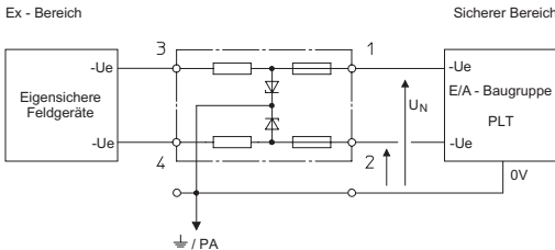
Zwei-Kanal-Sicherheitsbarrieren Potential: - / -
