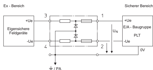
Zwei-Kanal-Sicherheitsbarrieren Potential: + / -
