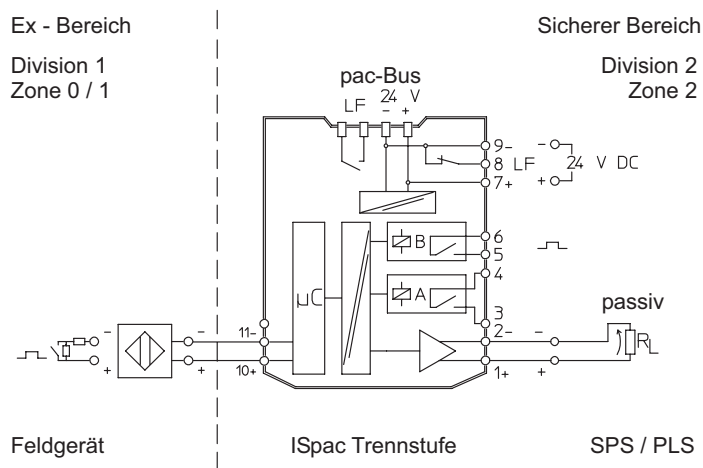
Anschlussplan 9146/10-11-12
