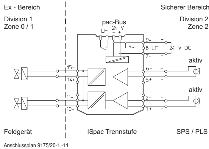
Anschlussplan 9175/20-1-11
