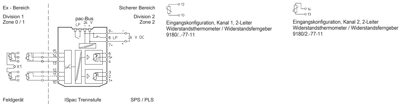
Anschlussplan 9180/2.-77-11
