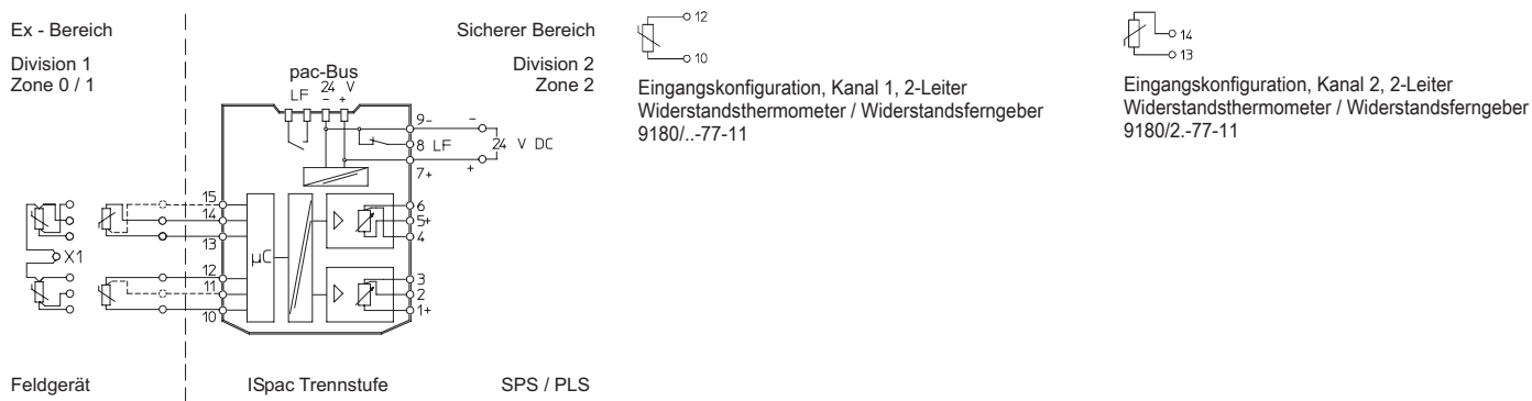
Anschlussplan 9180/2.-77-11
