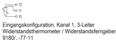
Anschlussplan 9180/2.-77-11
