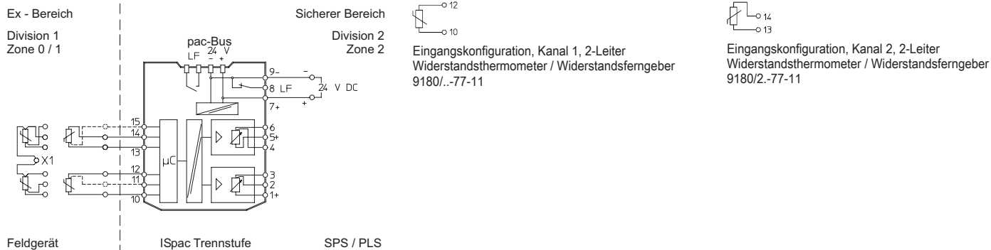
Anschlussplan 9180/2.-77-11
