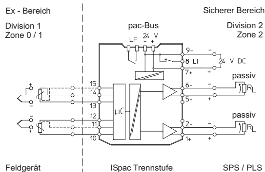
Anschlussplan 9182/20-51-11
