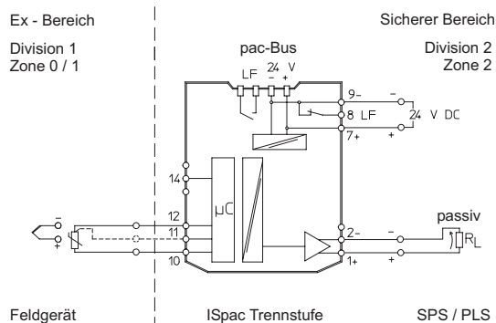
Anschlussplan 9182/10-51-11; 9182/10-51-13
