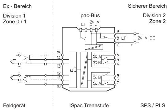
Anschlussplan 9182/20-50-12
