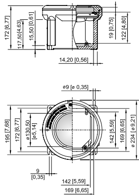
Gehäuse Größe 3 mit Schauglas
