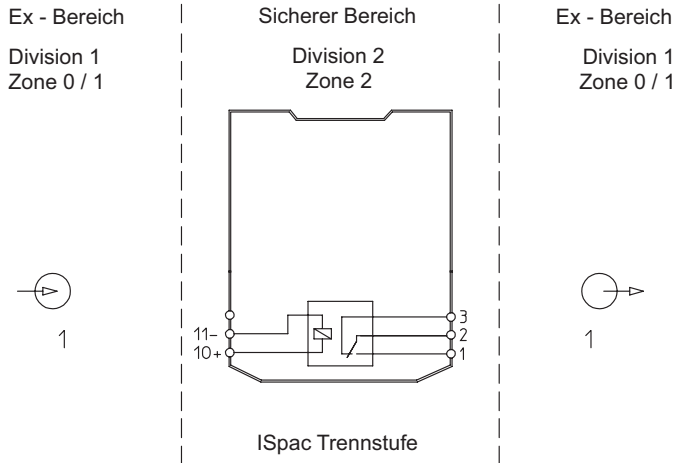
Anschlussplan 9172/12-11-00
