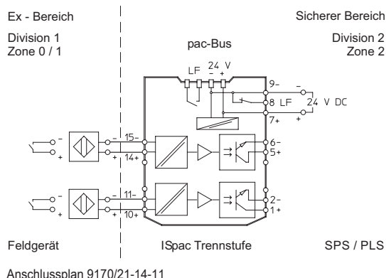
Anschlussplan 9170/21-14-11
