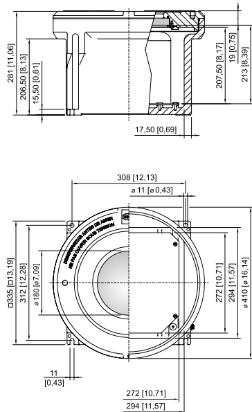
Gehäuse Größe 6 mit Schauglas
