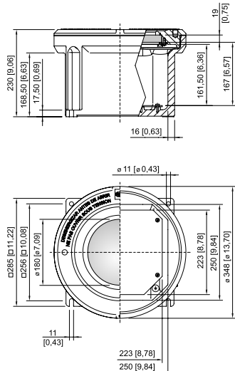
Gehäuse Größe 5 mit Schauglas
