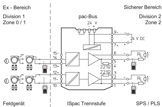
Anschlussplan 9160/23-10-10
