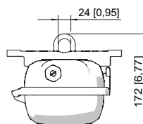
Montagebügel montiert in Montageschiene
