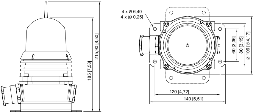
Mazeichnung (alle Mae in mm [Zoll]) – nderungen vorbehalten
