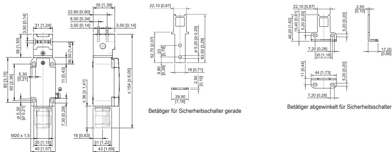
Sicherheitsschalter 8074/2--AZ-20
