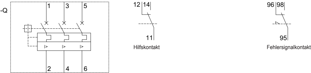
Geräteschaltplan
