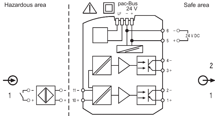
Anschlussbild 9270/11-19-15
