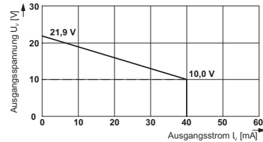
Ausgangskennlinie 9276/10-21-40
