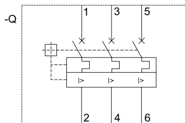
Geräteschaltplan
