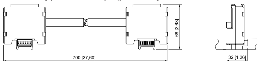
BusRail Verlängerung
