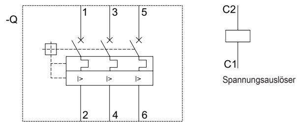
Geräteschaltplan
