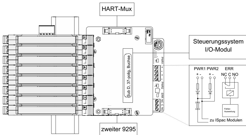
Anschlussbild 9295/12H2-XX0-08A5
