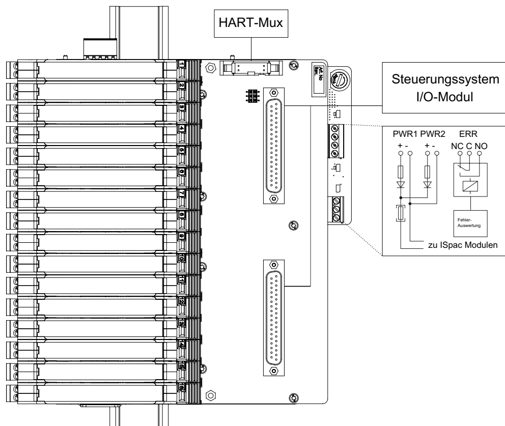
Anschlussbild 9295/22H2-XX0-08B3
