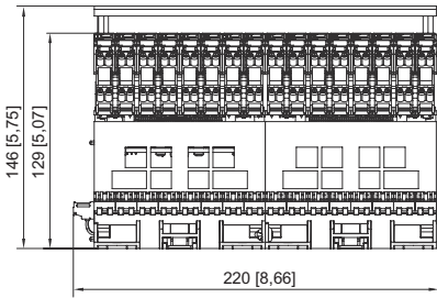
pac-Träger 16 slots
