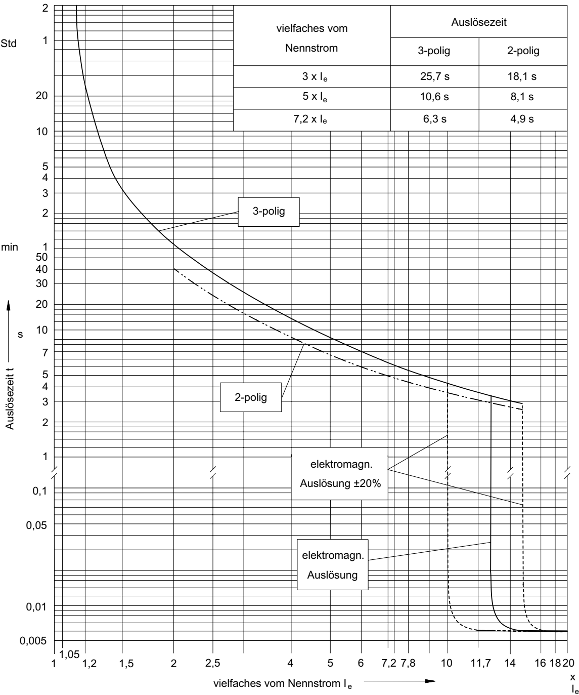
Auslösekennlinie 2,5 ... 4 A
