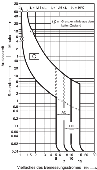
Auslösecharakteristik C
