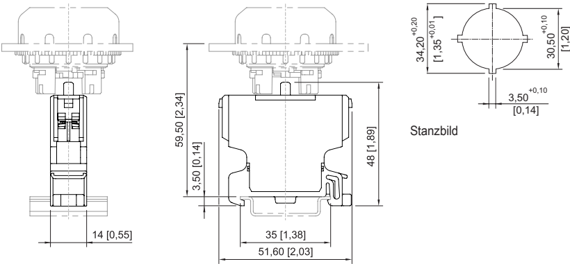
Kontaktelement für Tragschienenmontage
