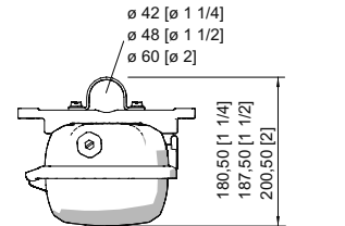
Rohrschelle montiert in Montageschiene
