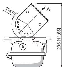
Wandbefestigungswinkel montiert in Montageschiene
