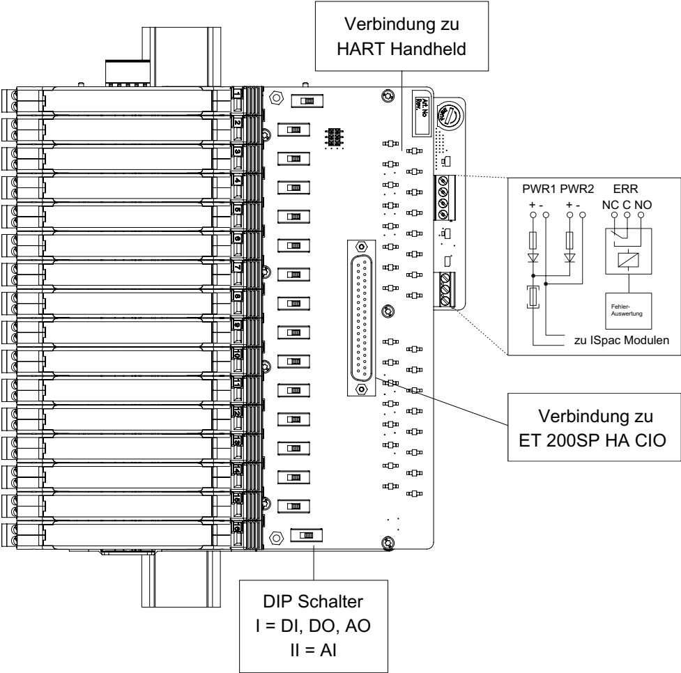
Anschlussbild 9295/21AH-SI3-01A5
