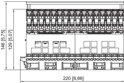
pac-Träger 16 slots
